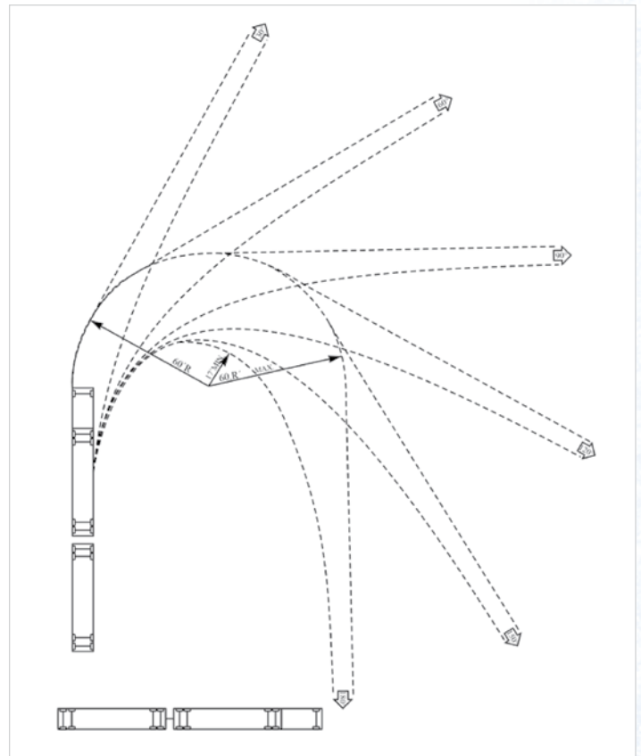
Рис. 1. Расчетная схема WB-114
